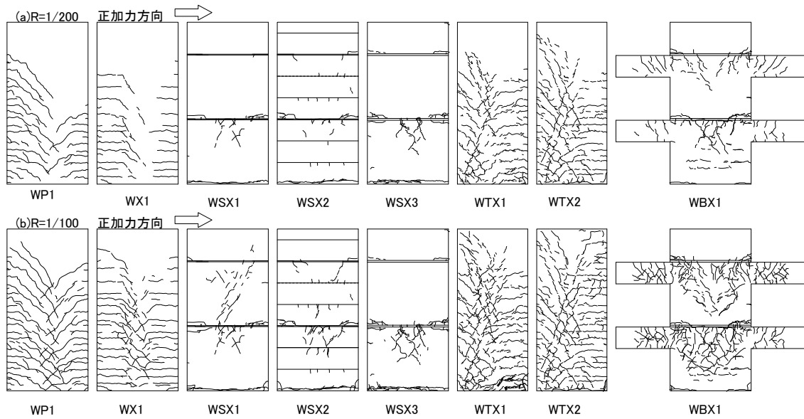
図4 損傷状況
