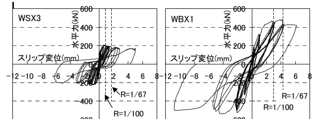
図 7 スリップ性状
