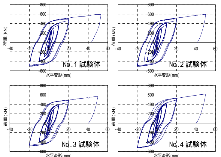
図 4 荷重 - 水平変形関係
