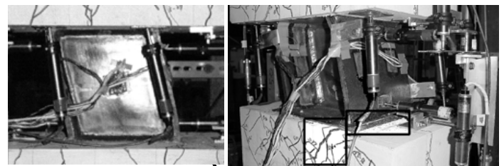
写真 1 ひび割れ状況( R=1/100 )
