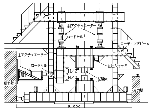
図3 加力装置
