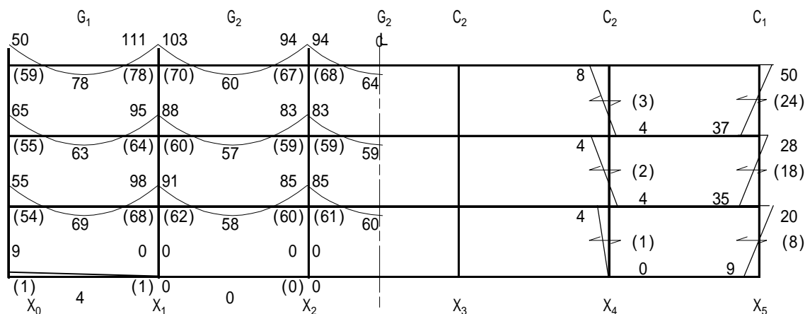
図 - 2 鉛直荷重時ラーメン応力分布 2) Y 0 , Y 3 ラーメン
