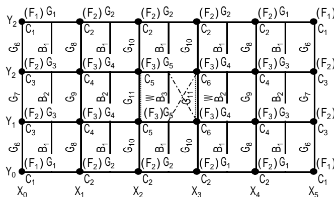
記号 G:大梁 B:小梁 C:柱 W:耐震壁 F:基礎
