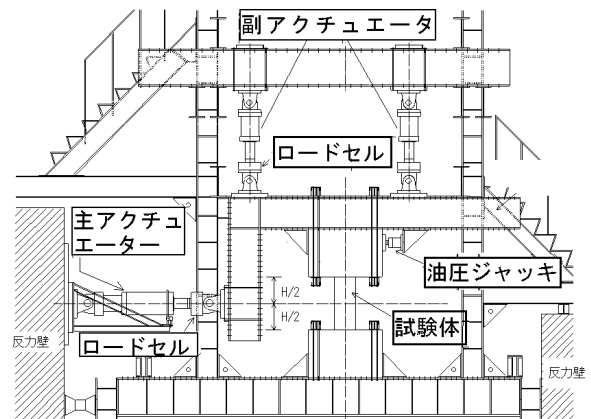
図 3 加力装置
