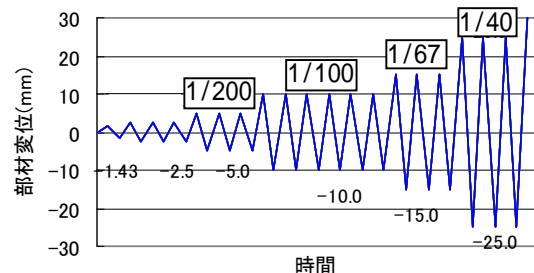
図 4 加力サイクル
